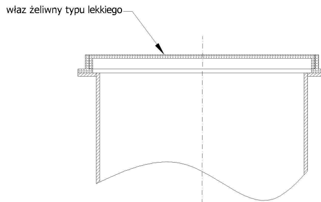
Zwieńczenie separatora włazem żeliwnym typu lekkiego
