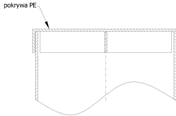
Zwieńczenie separatora włazem z tworzywa sztucznego (PEHD)
