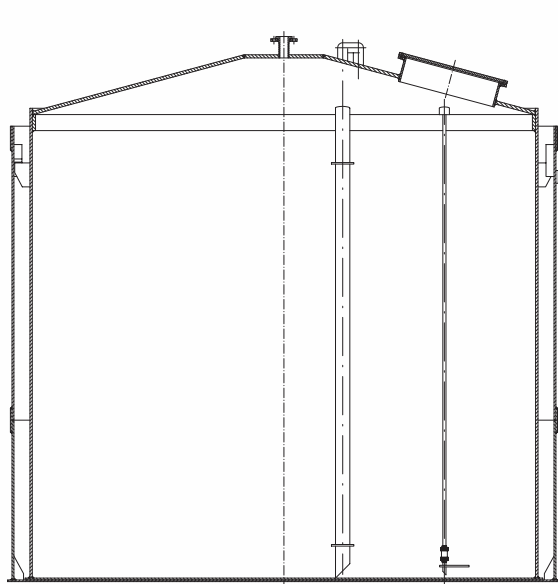
Zbiornik na media żrące z wanną wychwytyjącą - rysunek poglądowy.
